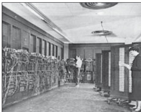
ENIAC
